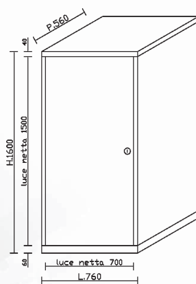
ARMADIO LOCALE MACCHINE STANDARD PER CORSE da 10.500 mm a 16.000
