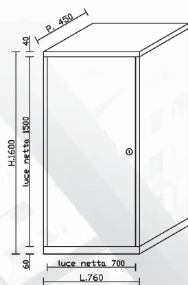
ARMADIO LOCALE MACCHINE STANDARD PER CORSE FINO 10.500 mm
